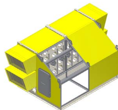
Рис. №5 КВОУ на расход воздуха 80000 м 3 /ч с фильтрующими элементами Donaldson GDH.
